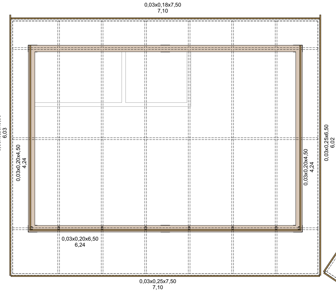
TÁBUAS DE FECHAMENTO ESCALA: 1:50
