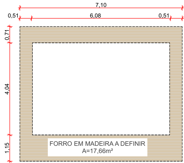
FORRO ESCALA: 1:100
